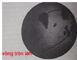
Hình 2.8: Đường trắc địa trên mặt trái đất chính là vòng tròn lớn và nó là đường ngắn nhất giữa hai điểm trên mặt đất.
