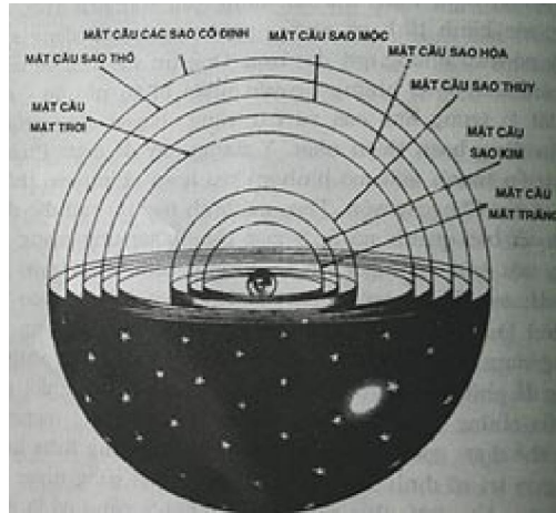
Hình 1.1: Mô hình vũ trụ của Aristotle - Ptolemy coi trái đất là trung tâm của vũ trụ.
