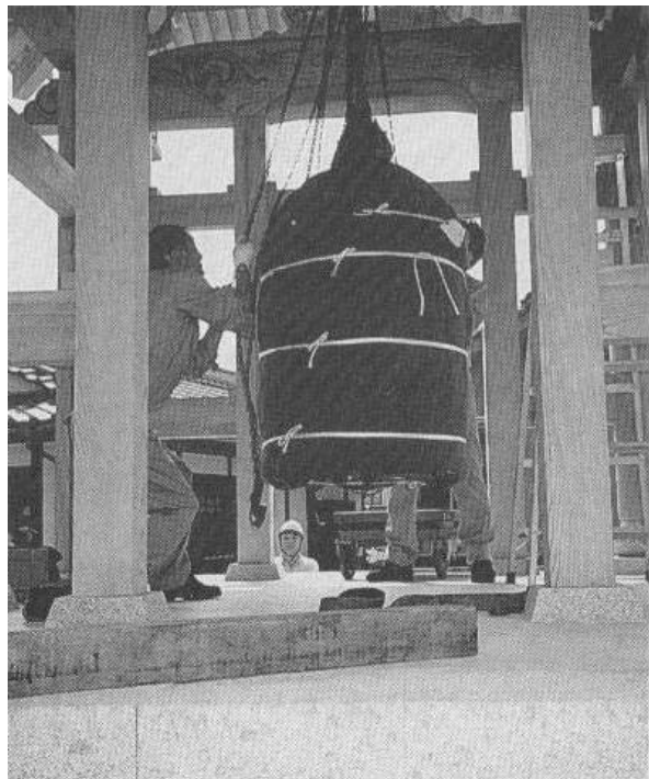
梵鐘取付
